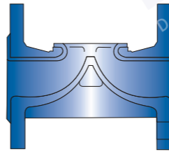
DIN PATTERN
