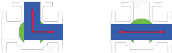
T 型三通球阀 NO.4
