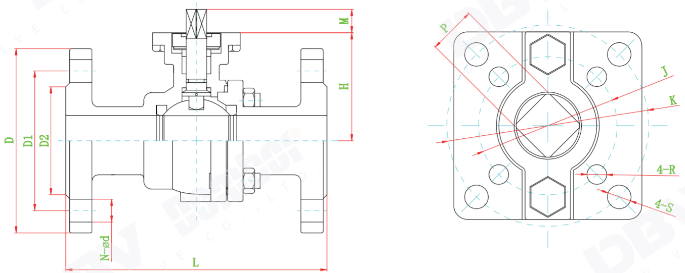
GB PN16~40 主要外形尺寸表 Main dimensions table
