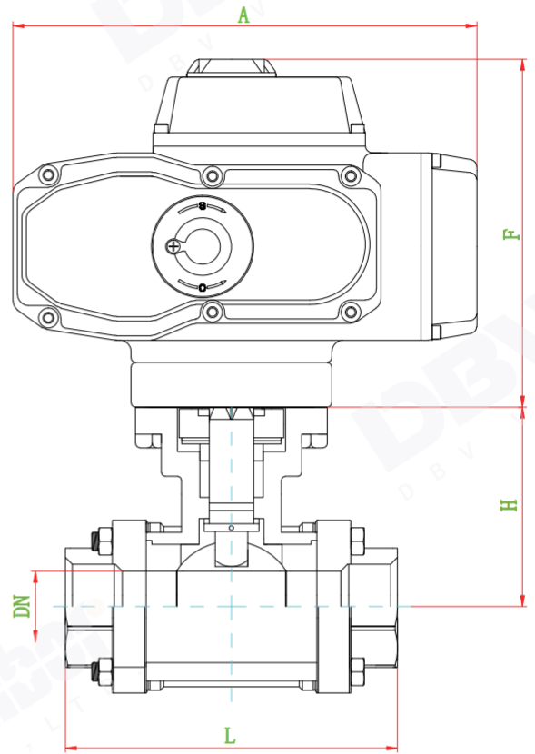
电动螺纹球阀
