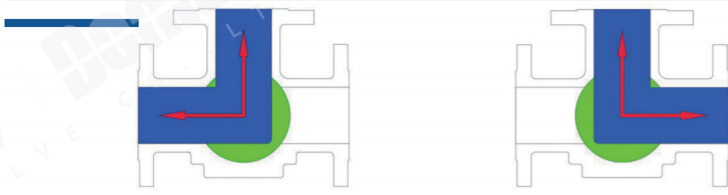
L 型三通球阀
