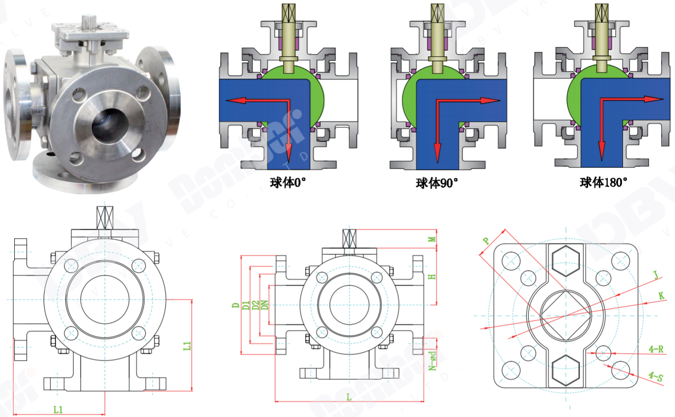
GB PN16 主要外形尺寸表 Main dimensions table
