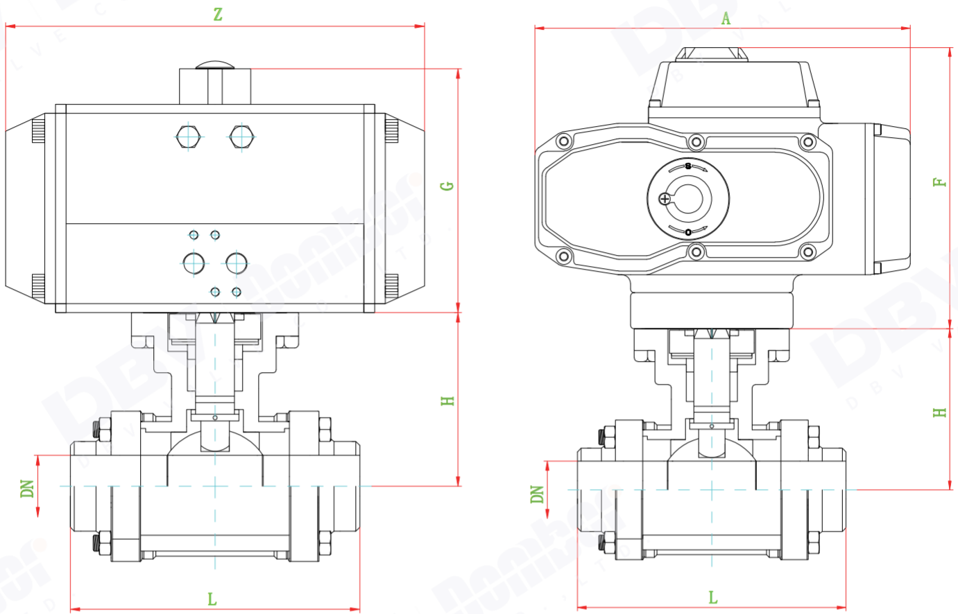
电动对焊球阀
