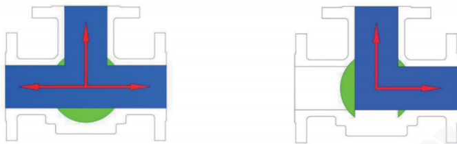
T 型三通球阀 NO.3
