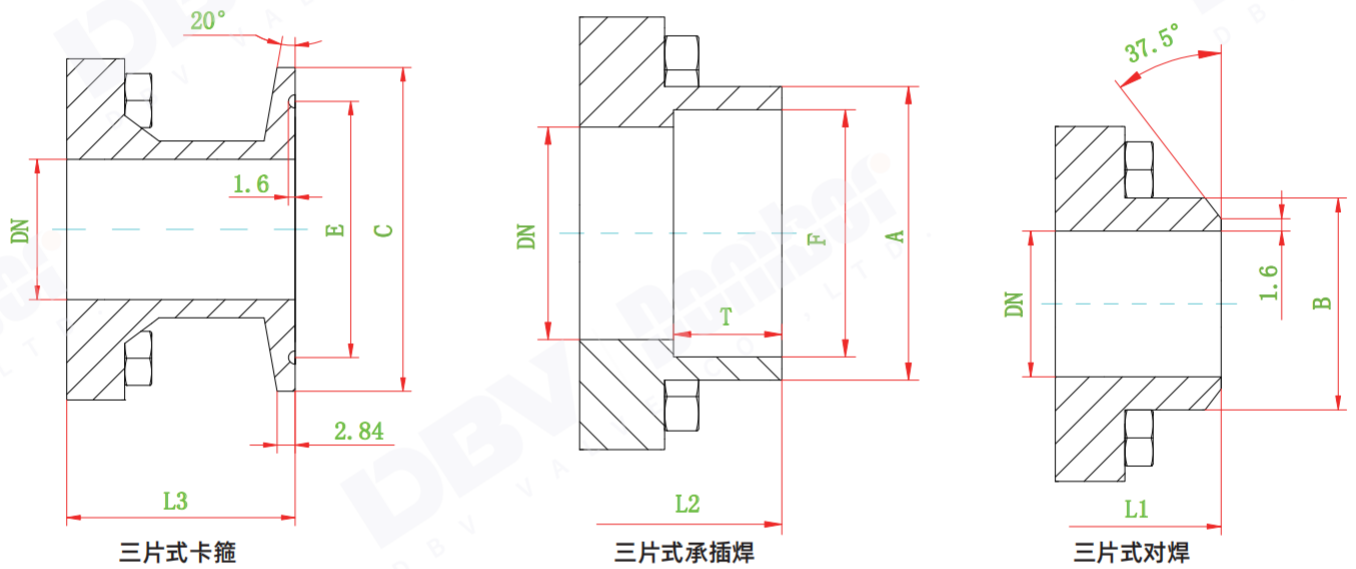
1000WOG 主要外形尺寸表 Main dimensions table
